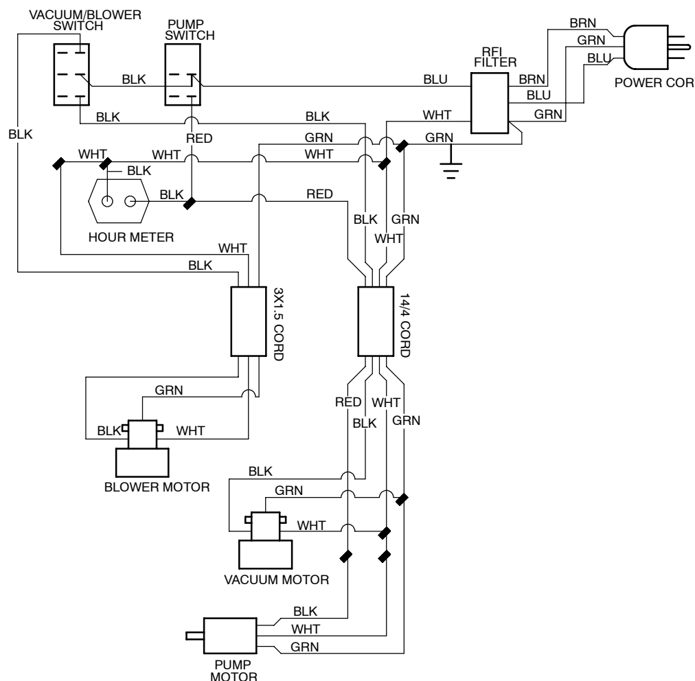
220V/230V/240 WIRING DIAGRAM DIAGRAMA DE CABLEADO DIAGRAMME DE CÂBLAGE
