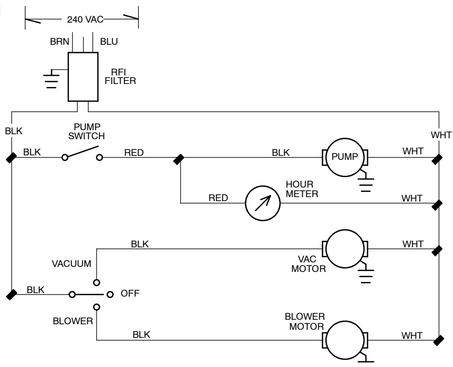
220V/230V/240 LADDER DIAGRAM DIAGRAMA ESCALONADO DIAGRAMME D'ÉCHELLE
