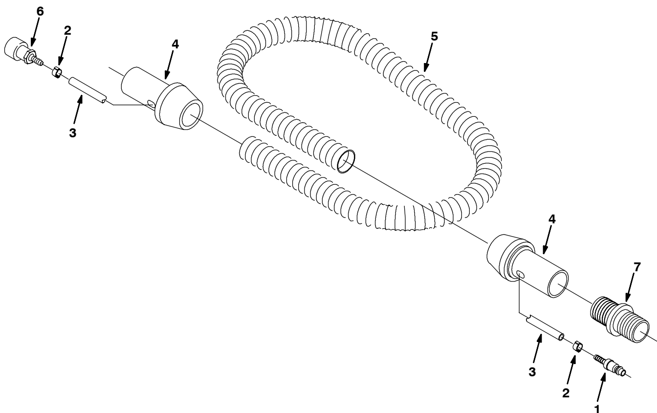
Fig. 3 - Power Wand Hose Assembly - Handschrubbschlauch Gruppe - Groupe Tuyau flexible de la Laveuse à Main
