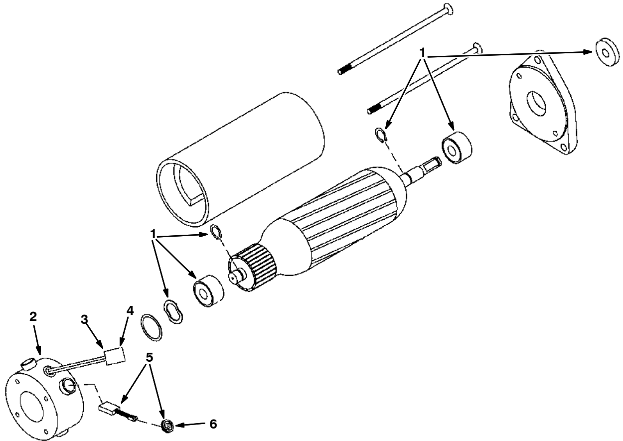
Fig. 3 - 374265AM- Transaxle Motor - Getriebe Motor - Moteur d'Instigateur
