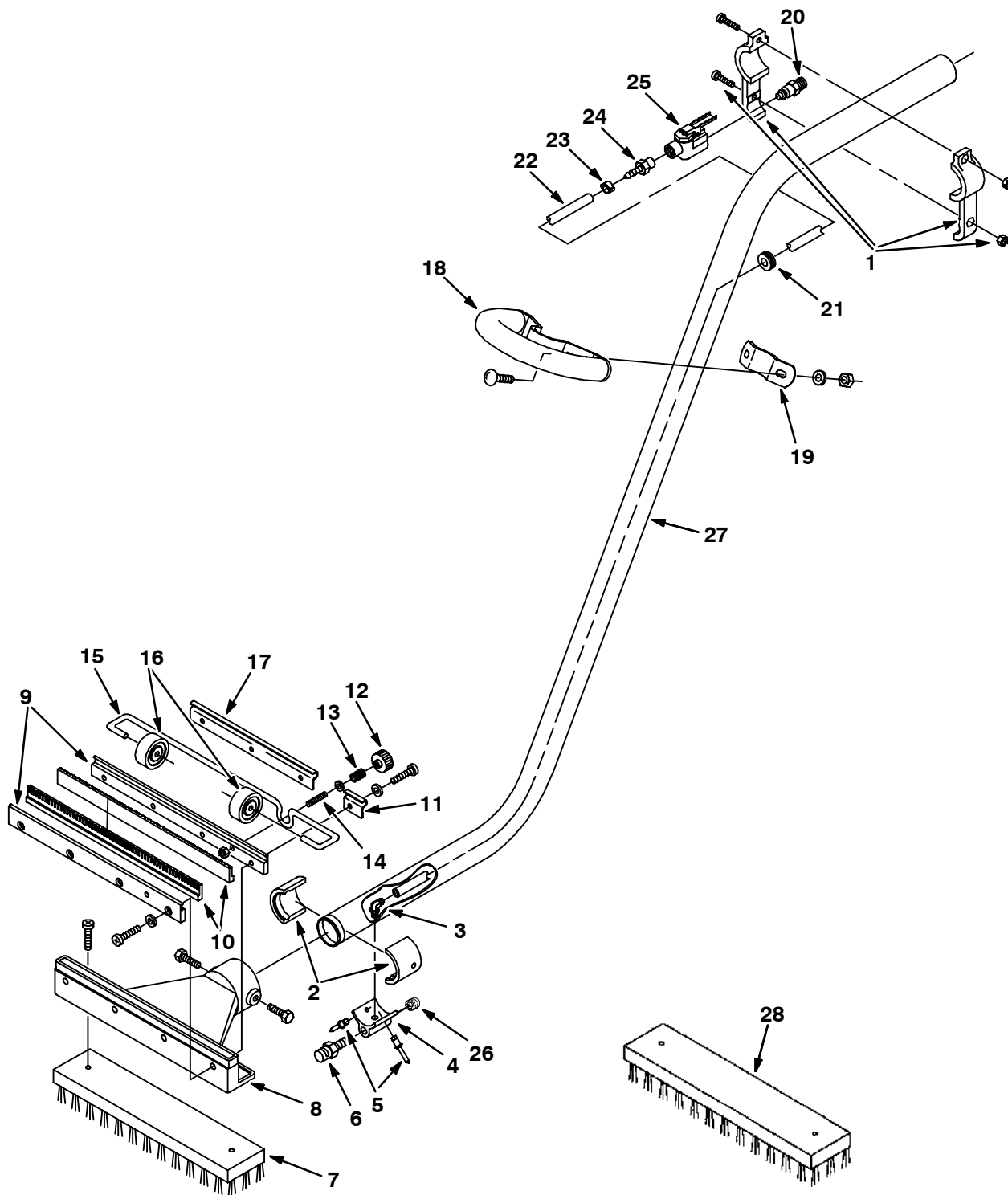
Fig. 4 - Power Wand Assembly - Handschrubbarm Gruppe - Groupe Laveuse à Main
