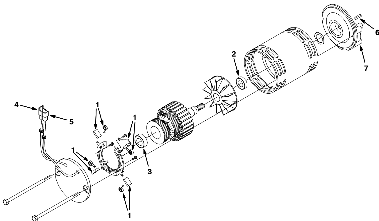
Fig. 8 - 222255AM - Electric Motor - Elektromotor - Moteur d'Électrique
