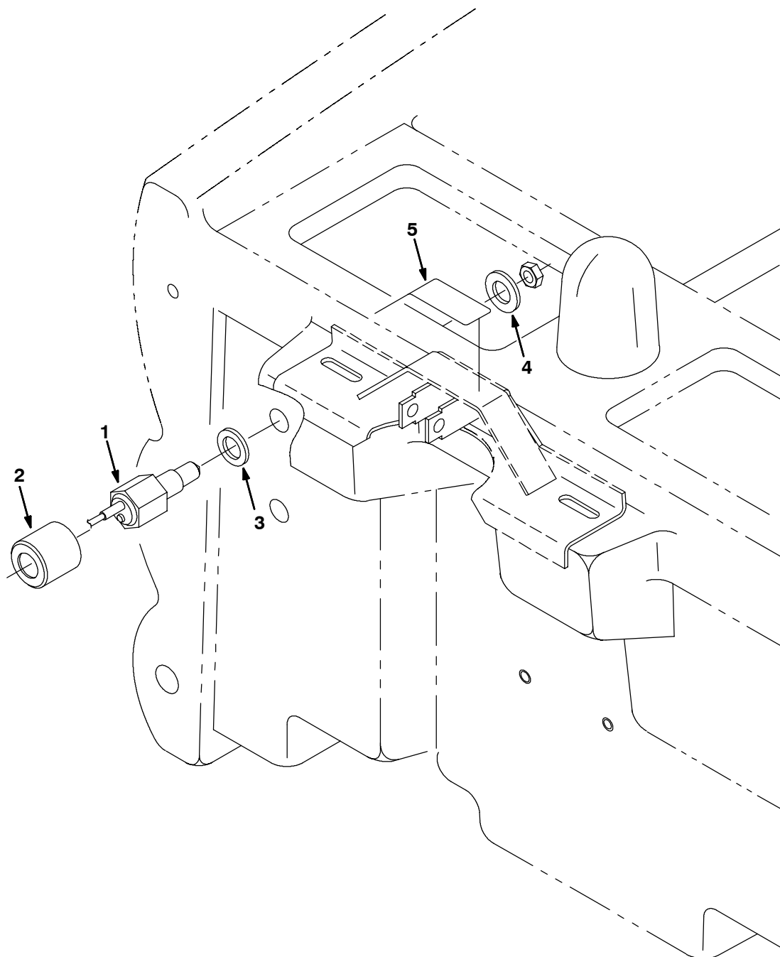
Fig. 20 - Optical Sensor Kit (57150 0001-xxxx) — Optischer Sensor-Satz (57150 0001-xxxx) — Jeu de pièces du capteur optique (57150 0001-xxxx)
