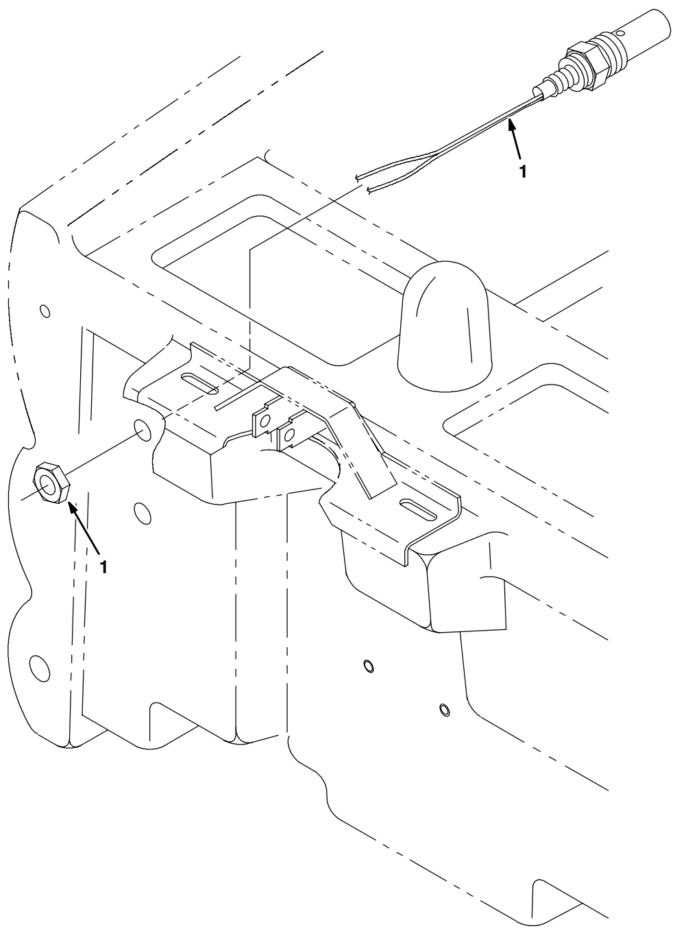
Fig. 21 - Shielded Sensor Kit — Abgeschirmter Sensor-Satz — Jeu de pièces détecteur blindé
