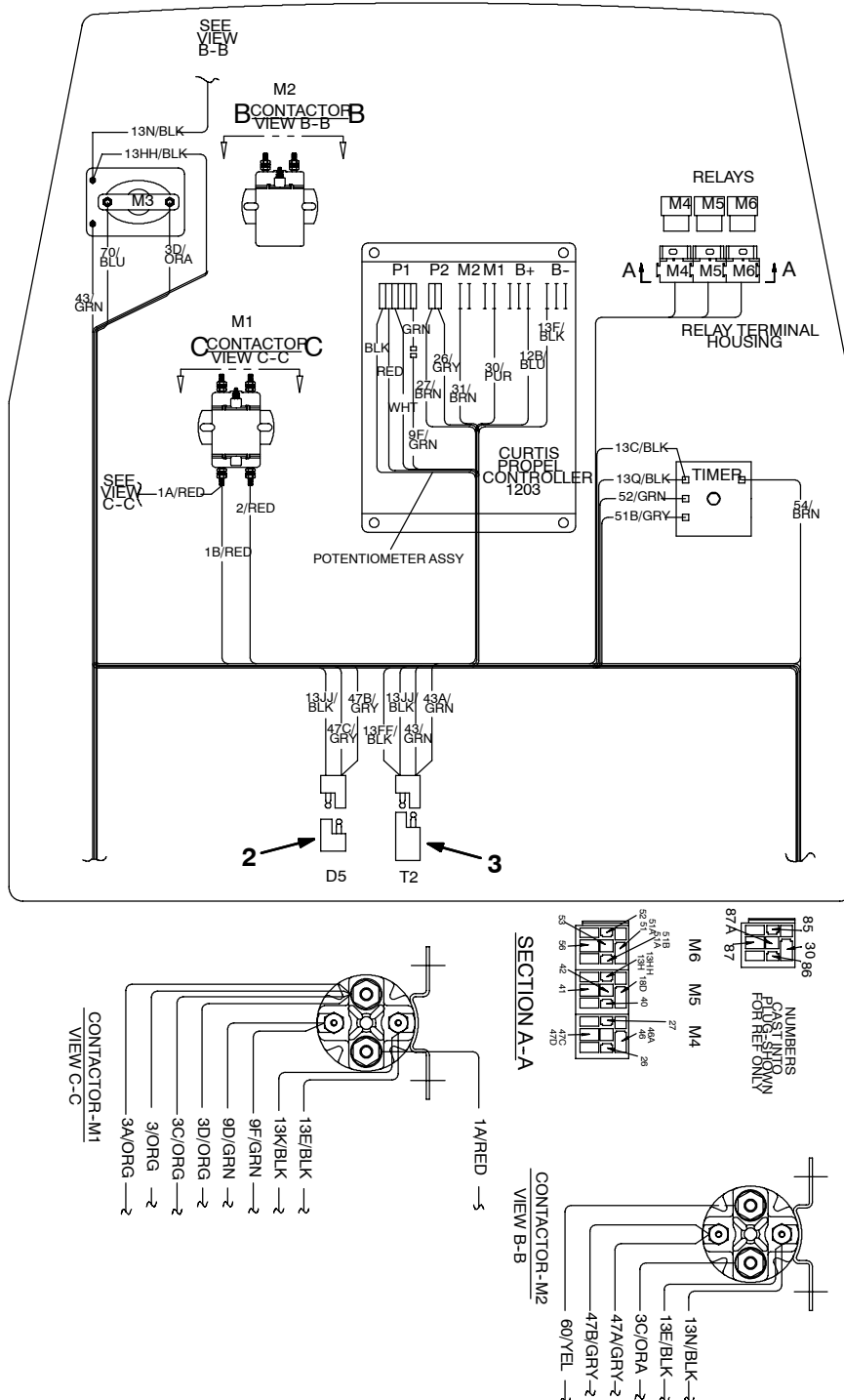
Fig. 39 - Wire Harness Group (57150 0001 - 57150 xxxx) - Kabelstrang Gruppe (57150 0001 - 57150 xxxx) - Groupe Faisceau de Fils (57150 0001 - 57150 xxxx)
