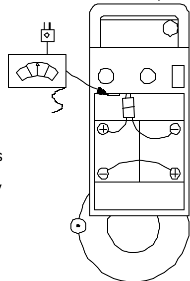
2 X 12 VOLT
