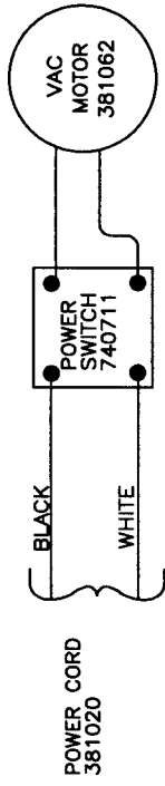
WIRING DIAGRAM 115 VOLT - MODEL C84790-00
