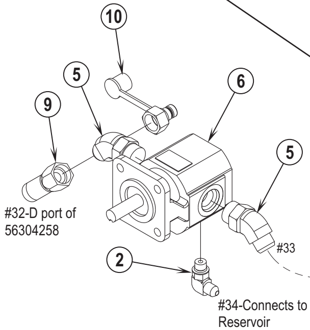
56304261 Squeeze Fan Motor Assy
